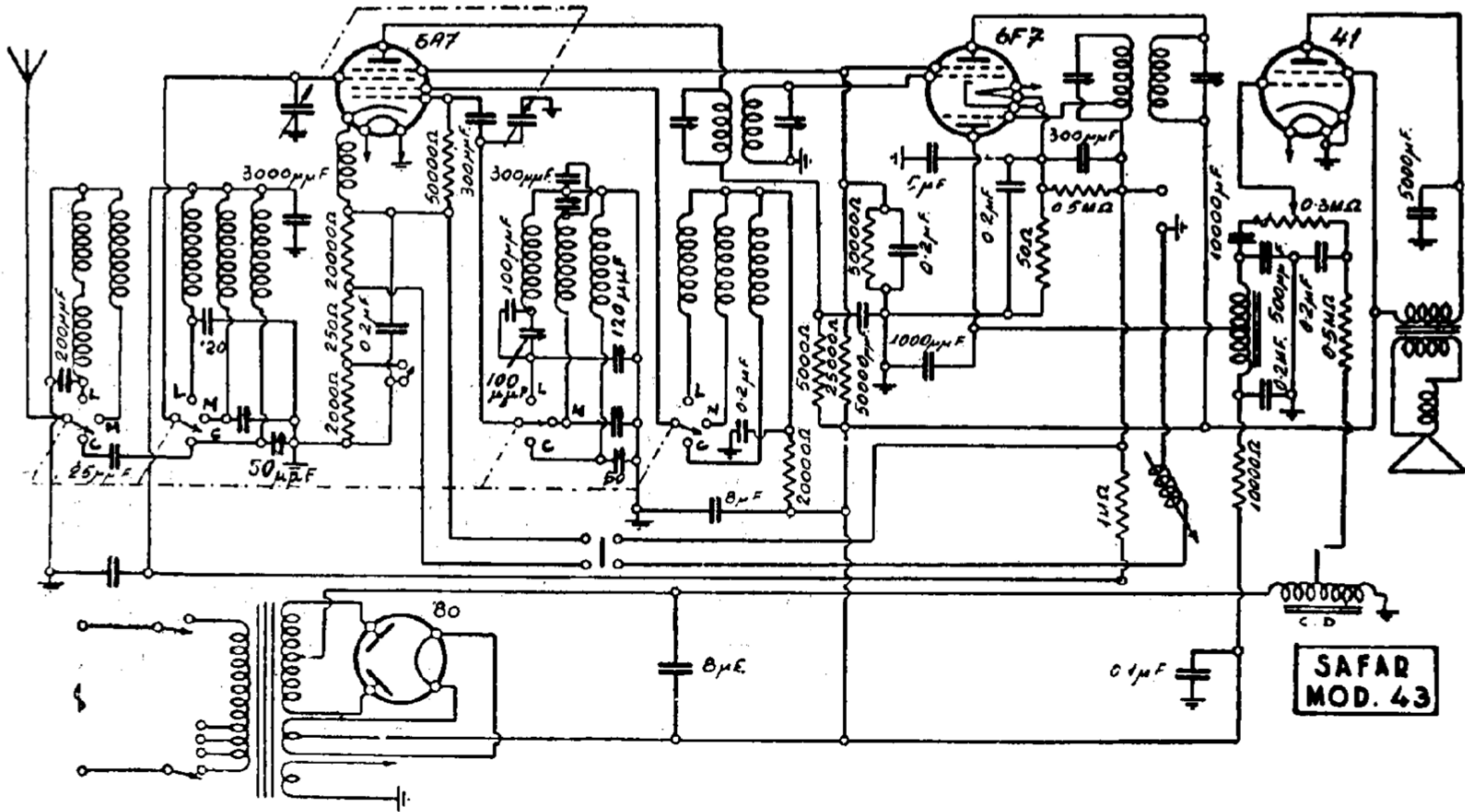
RADIO SAFAR. — Modello « 43 ». - Produzione 1935. - Media frequenza: 375 kc
